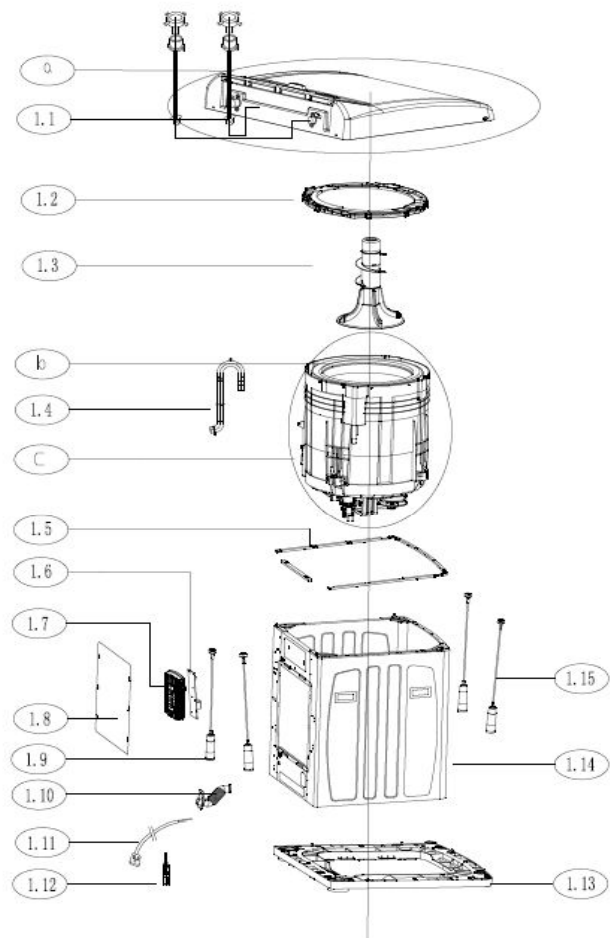
a: Top Cover Subassembly
