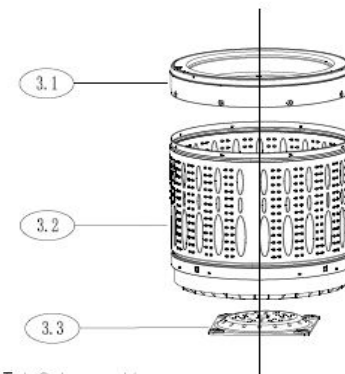
b: Spin Tub Subassembly
