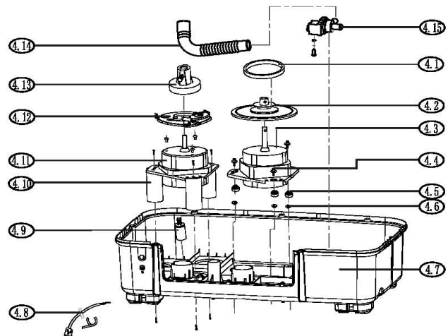
4:Base Subassembly
