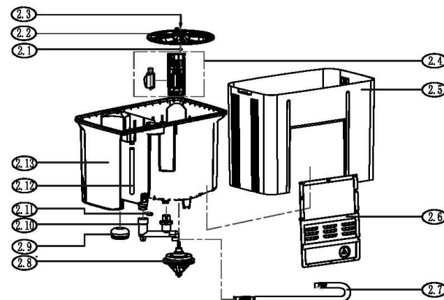
2:Cabinet Subassembly
