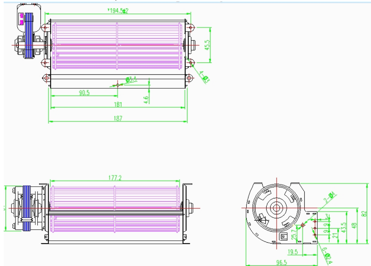
17471100000145 Fan Assembly
