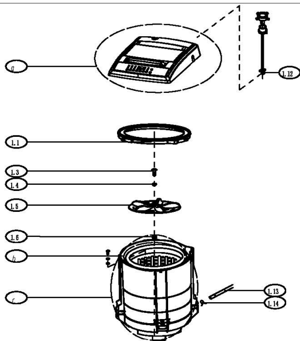
a: Top Cover Subassembly
