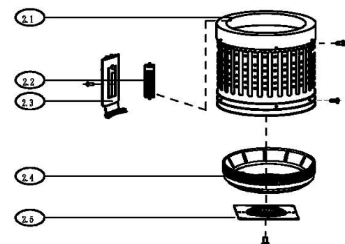
b: Spin Tub Subassembly
