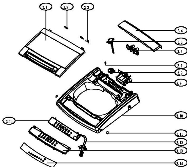
a: Top Cover Subassembly
