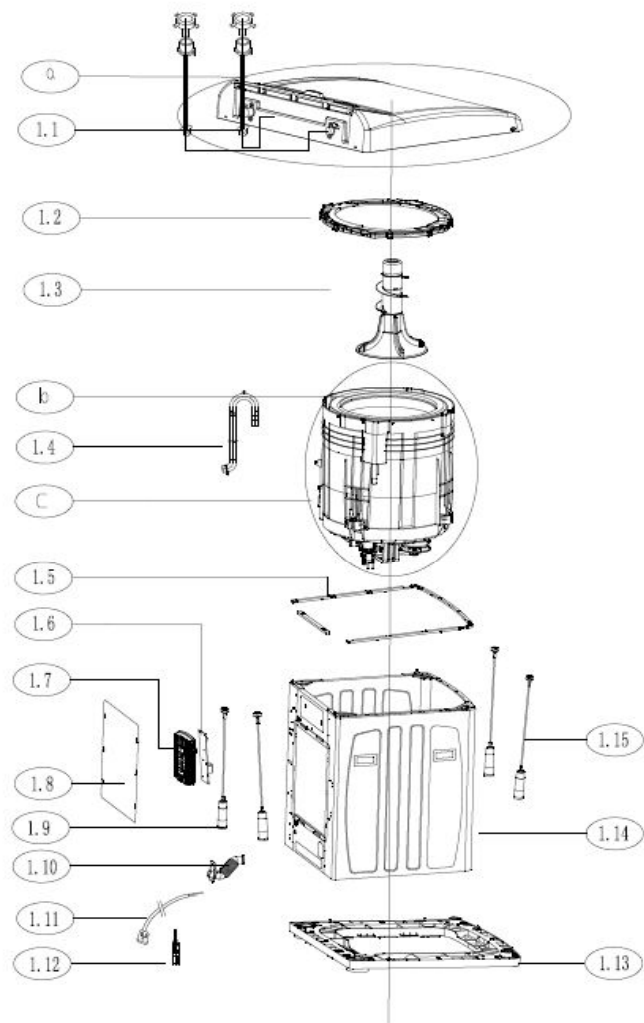
a: Top Cover Subassembly
