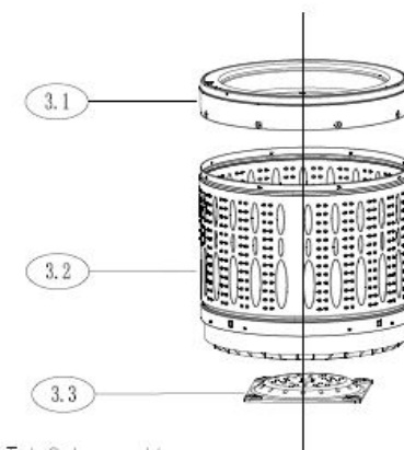
b: Spin Tub Subassembly
