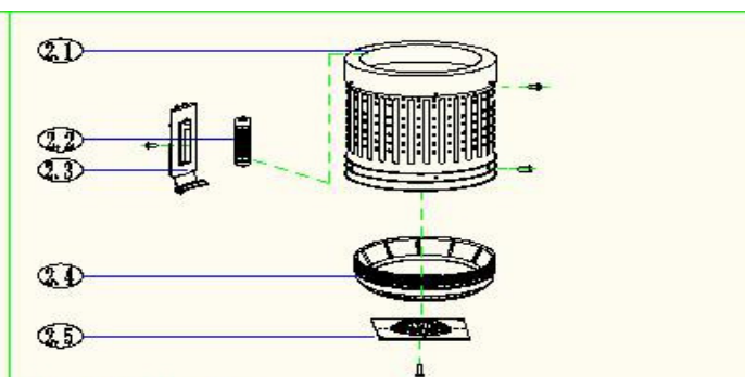
2-Spin Tub Subassembly
