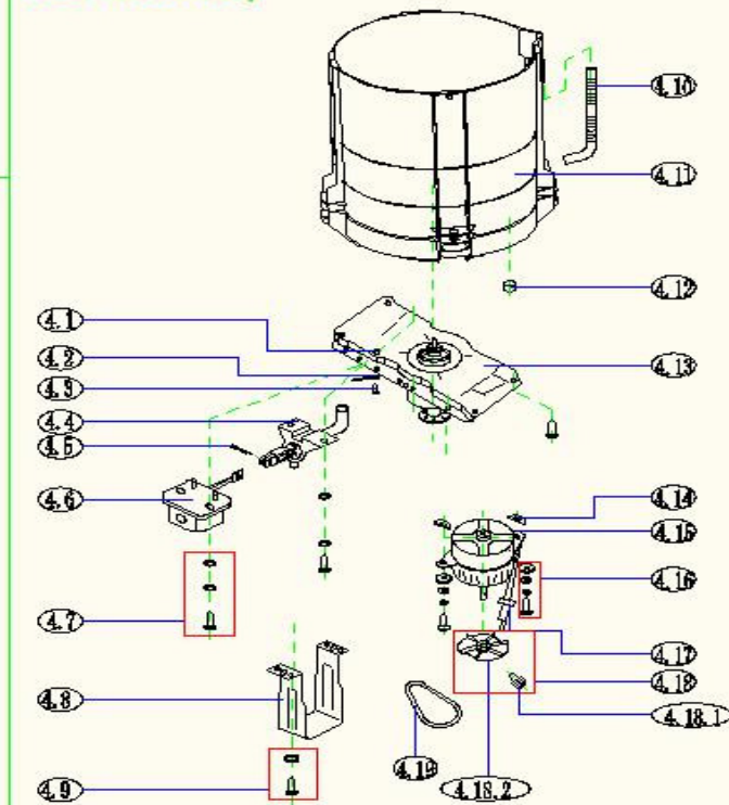
4-Outer Tub Subassembly
